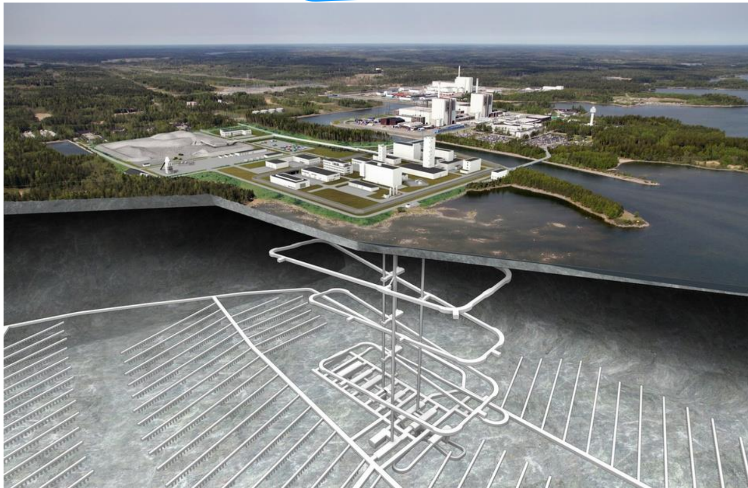
Giluminio atliekyno maketas. Paveikslėlio šaltinis: Karnbransleforvaret @Lasse Modin
