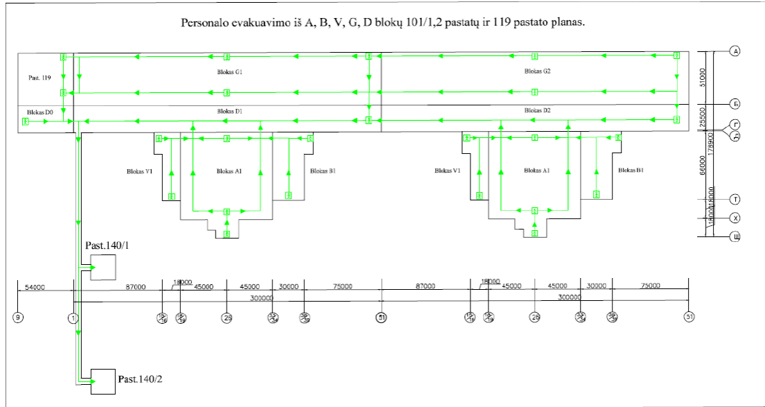
2 pav. Personalo evakuavimo iš 101/1,2 ir 119 pastatų A, B, V, G, D blokų planas
