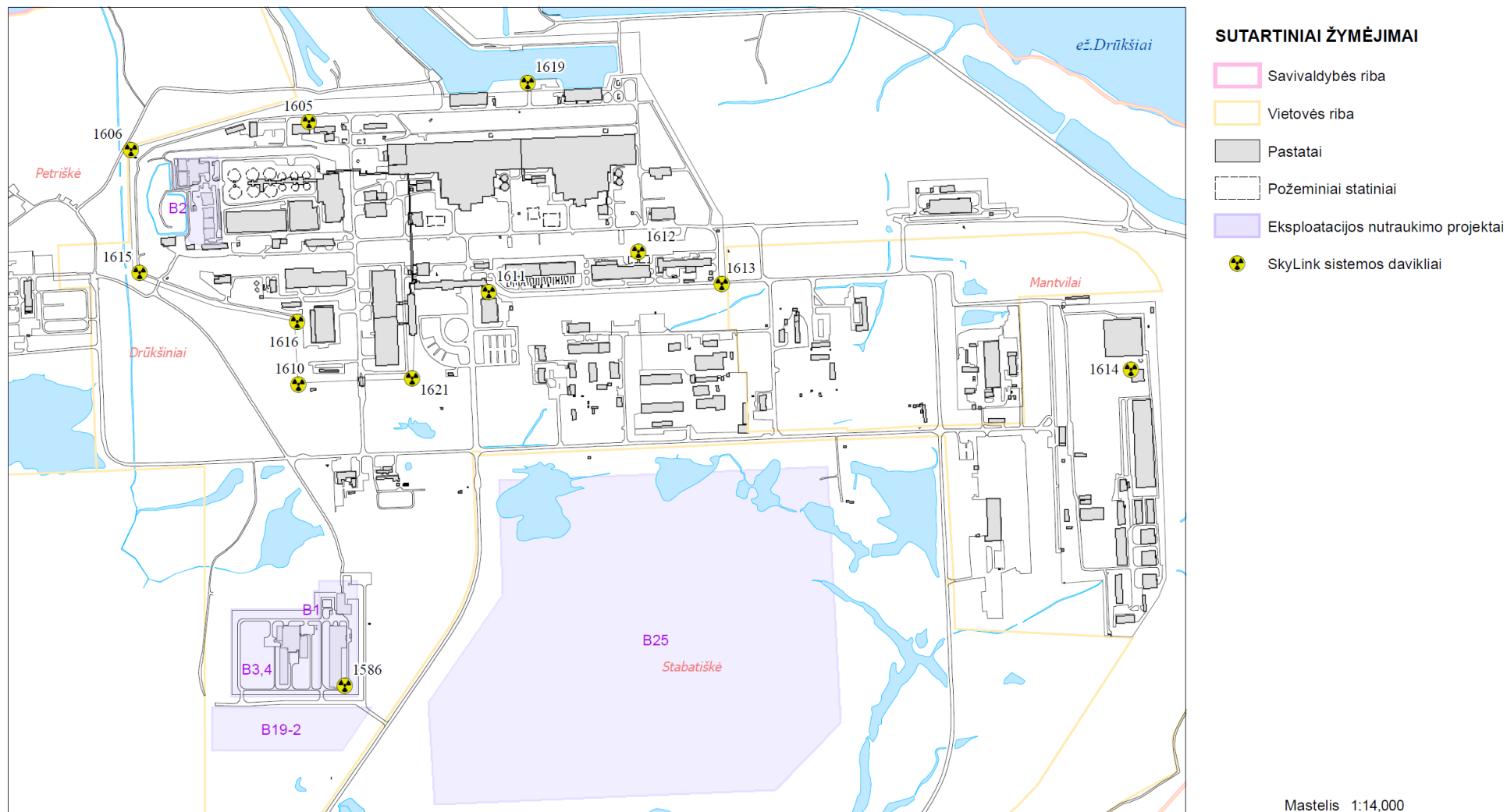
7.3-2 pav. „Skylink“ sistemos gama daviklių išdėstymas sanitarinėje apsaugos zonoje [8]
