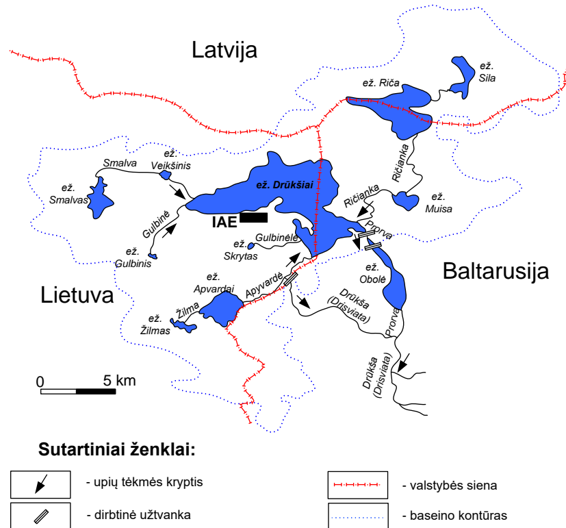
4.1-2 pav. Drūkšių ežero hidrografinio tinklo schema
