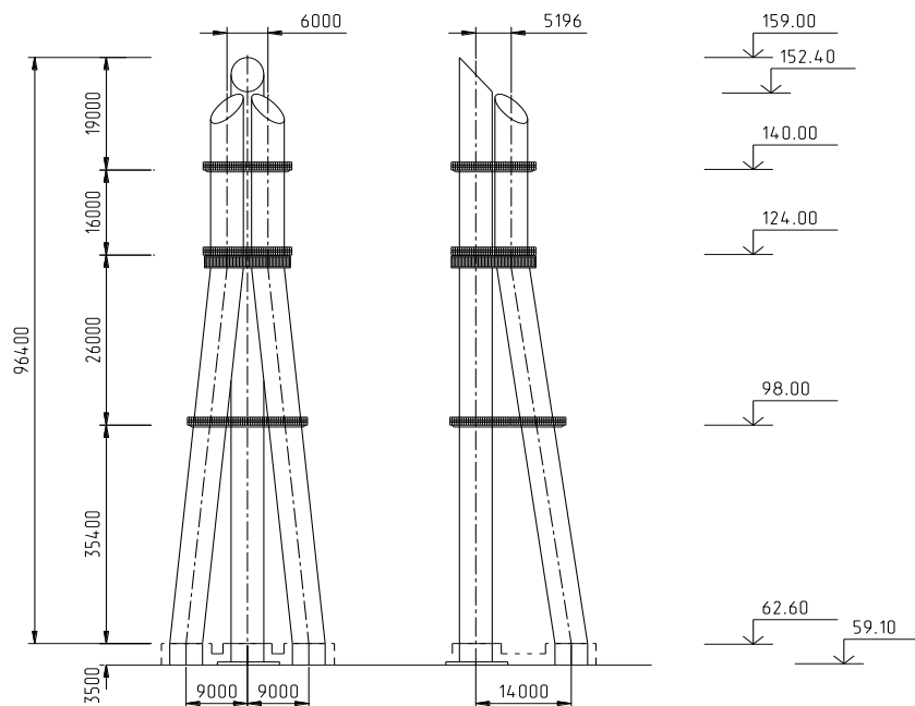
4.2-3 pav. 101/1,2 pastatų ventiliacijos vamzdžių schema
