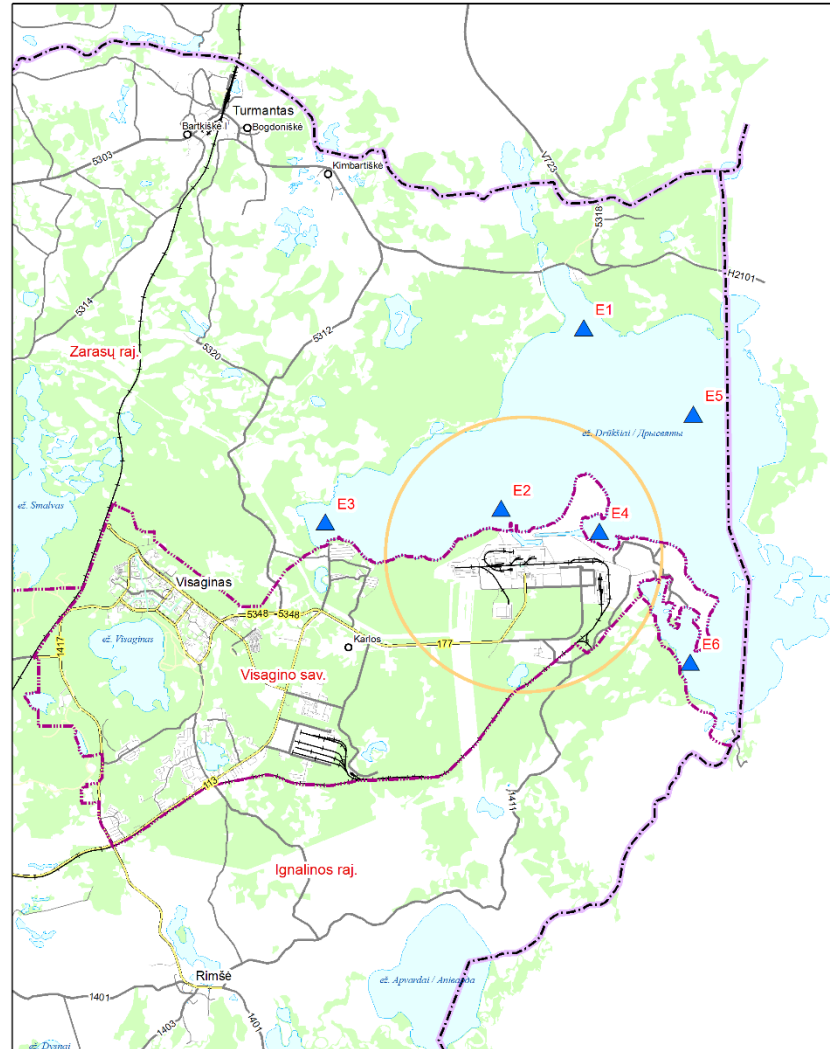
7.2-4 pav. „Nulinio“ fono tyrimo vietų išdėstymo schema Drūkšių ežere [8]
