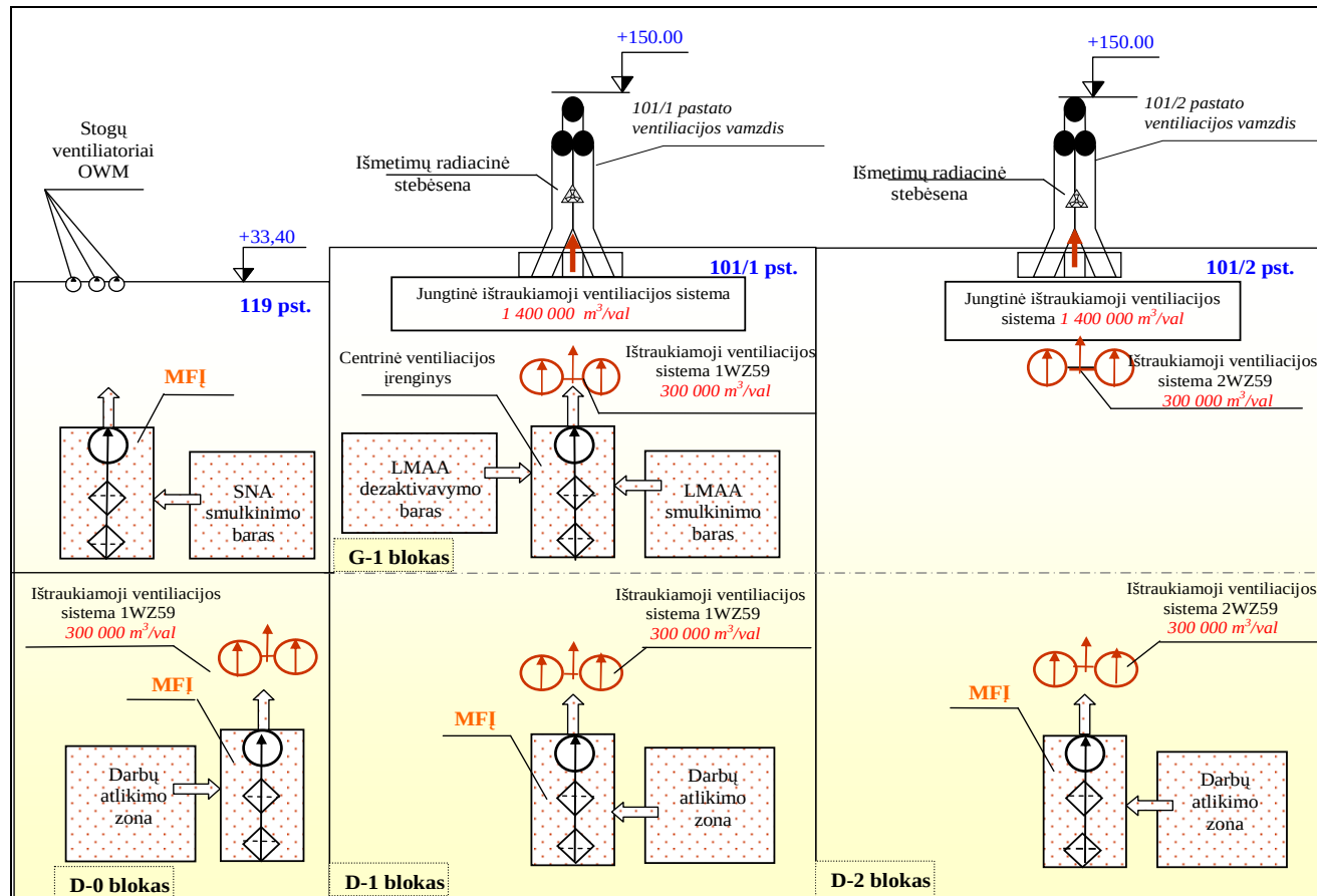
2.1.-1 pav. Principinė ventiliacijos organizavimo schema 2
