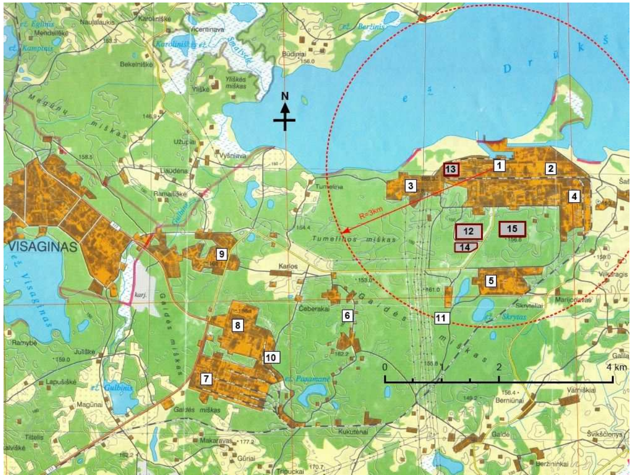
1.6-1 pav. Ignalinos AE SAZ ir šalia jos esantys objektai
