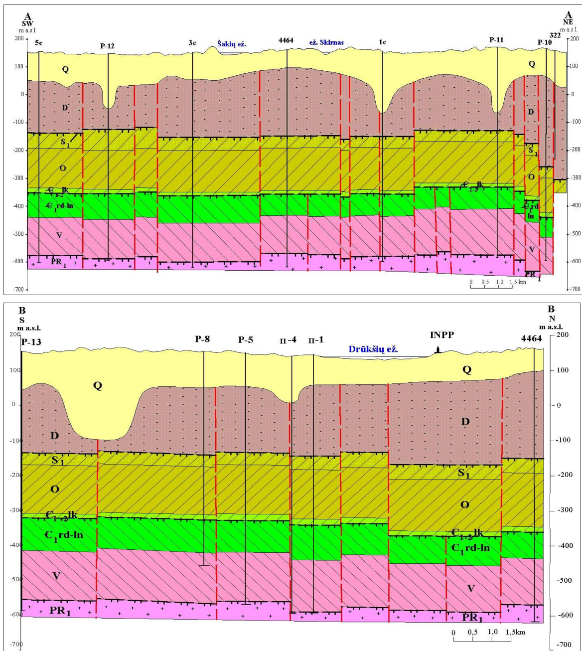
4.4.1-2 pav. IAE regiono geologiniai pjūviai [1] (pjūvių vietas žr. 4.4.1-3 pav.)
