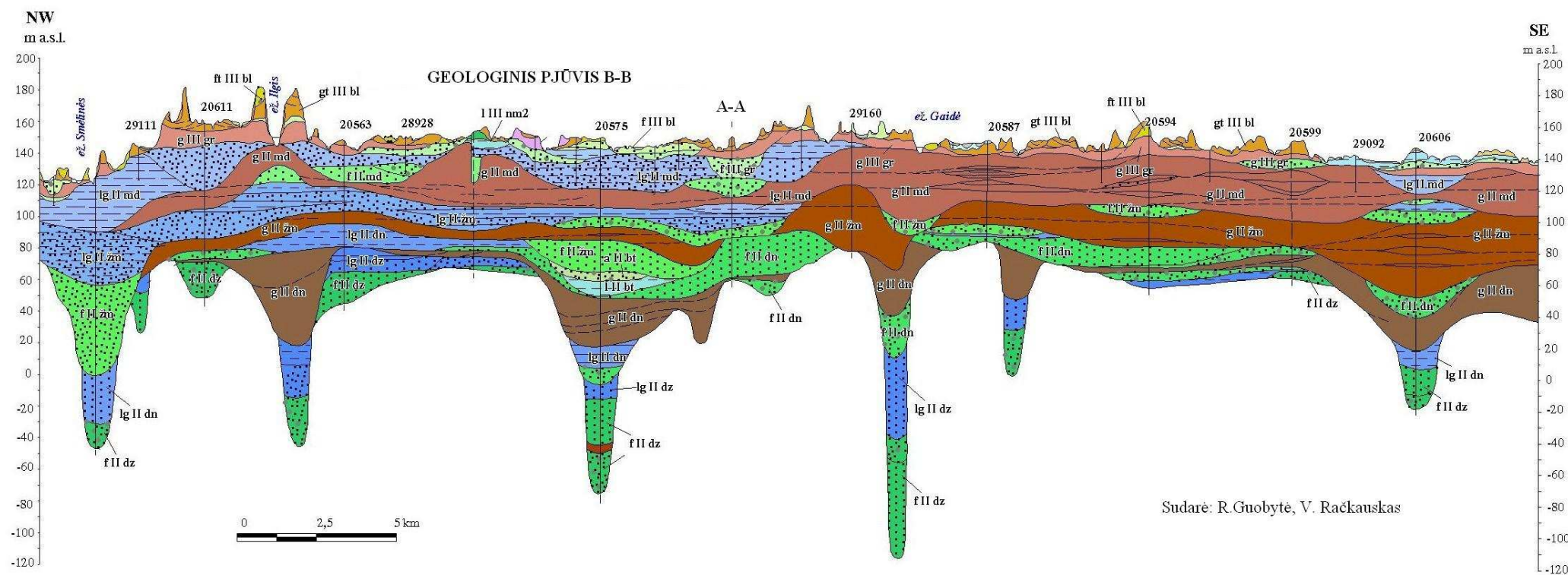
4.4.1.-6 pav. IAE regiono apylinkių kvartero geologinis pjūvis B-B (originalo mastelis 1:50 000, autoriai: R. Guobytė, V. Račkauskas [1]); legendą žr. 4.4.1-4 pav.
