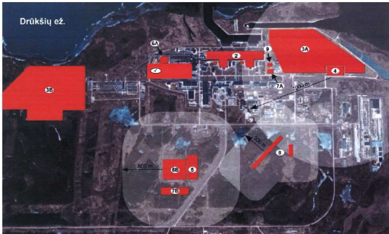
4.9.3-2 pav. IAE SAZ esantys ir planuojami BEO
