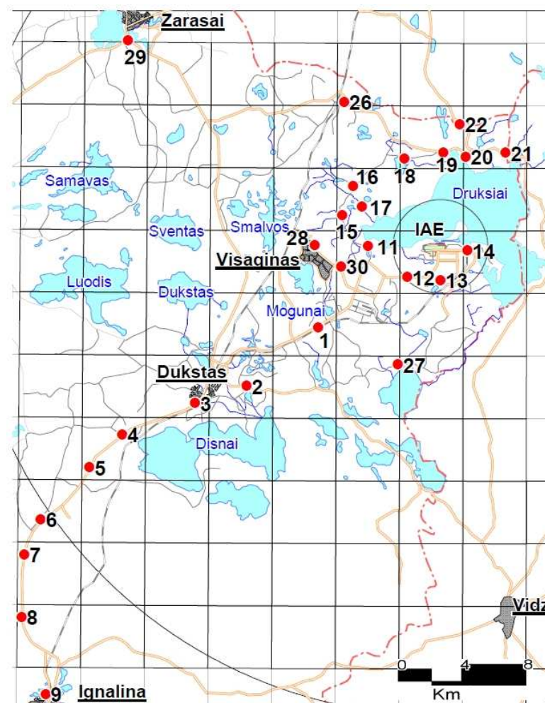
7.2.3-2 pav. TLD dozimetų išdėstymas [6]
