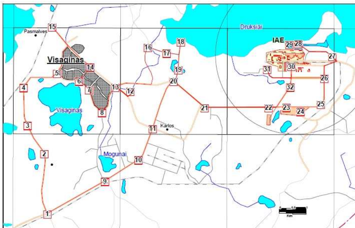
7.2.3-3 pav. „Skylink“ sistemos daviklių išdėstymas IAE perimetru [6]
