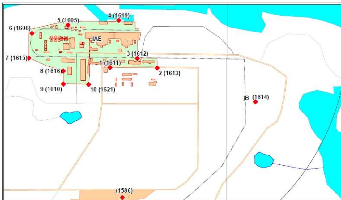
7.2.3-3 pav. „Skylink“ sistemos daviklių išdėstymas IAE perimetru [6]
