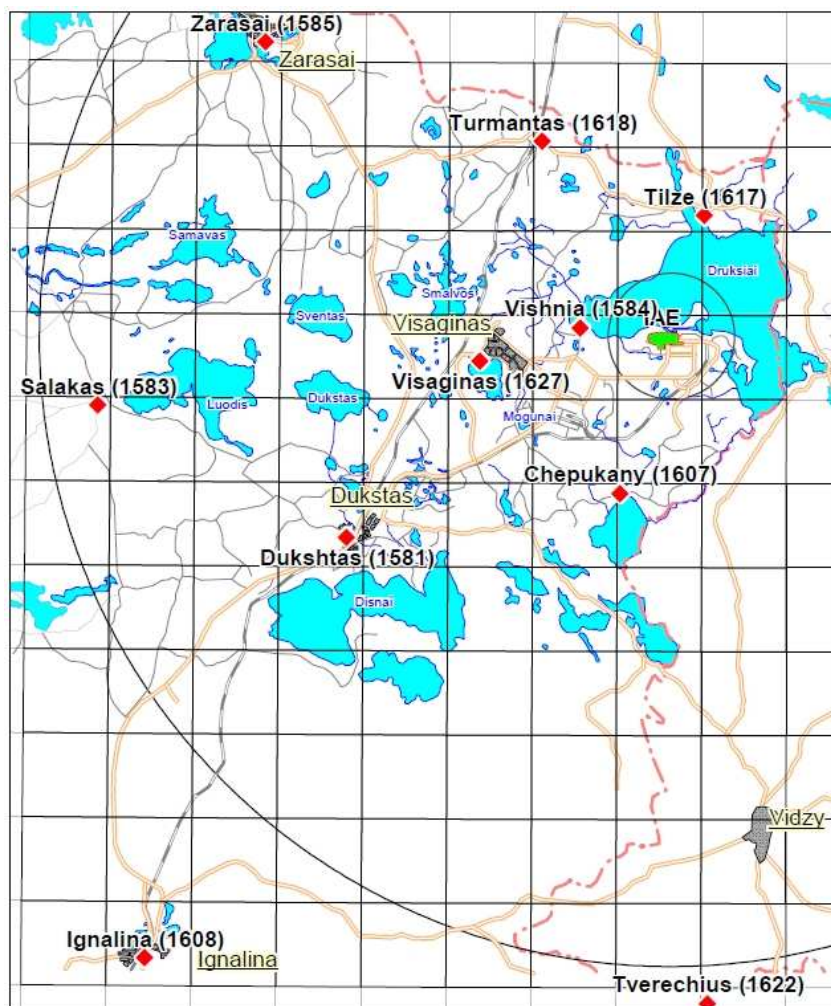
7.2.3-1 pav. „Skylink“ sistemos daviklių išdėstymas [6]
