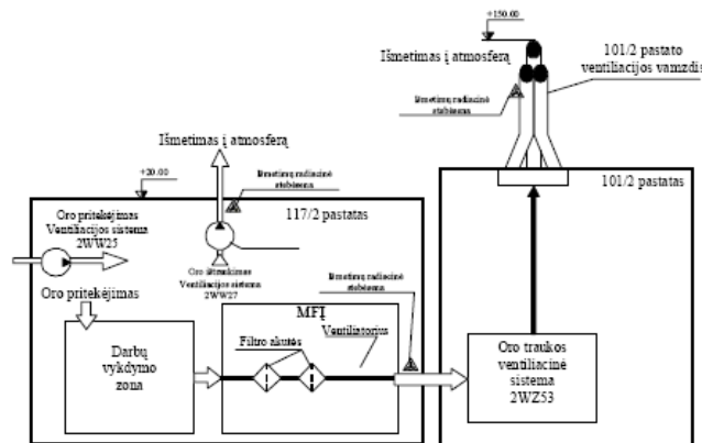
Principinė ventiliacijos organizavimo 117/2 pastate schema
