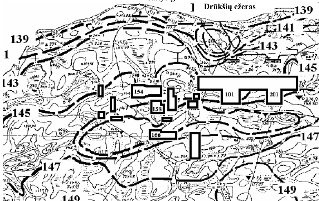
5-1 schema. IAE teritorijos absoliutinių gruntinio vandens lygių 1973 m. schema (prieš IAE statybą)
