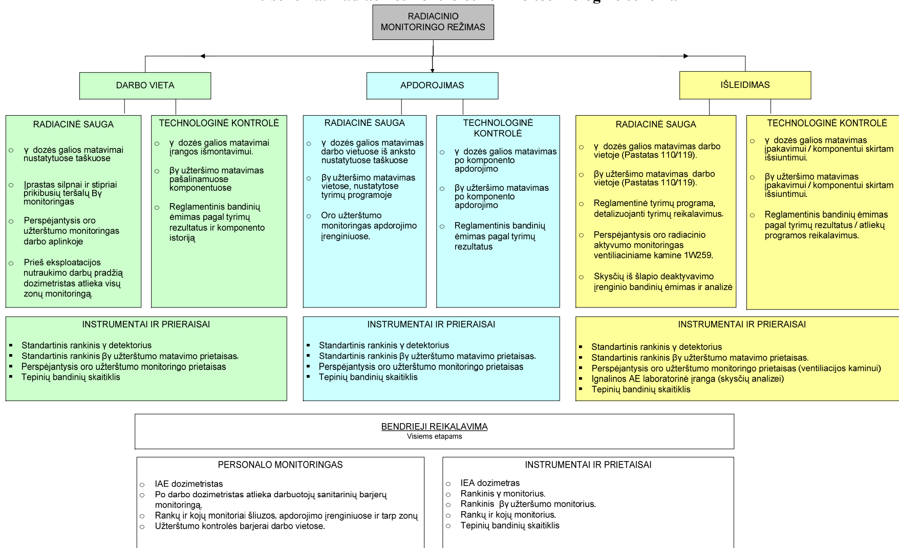
4-10 schema. Radiacinės kontrolės režimo technologinė schema
