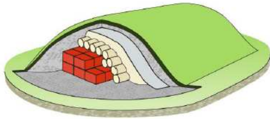
1.3-7 pav. Atliekų krovimo suprojektuotame LMAA atliekyne konceptualioji schema ir veikiančio Švedijos Oskarshamn AE atliekyno nuotrauka
