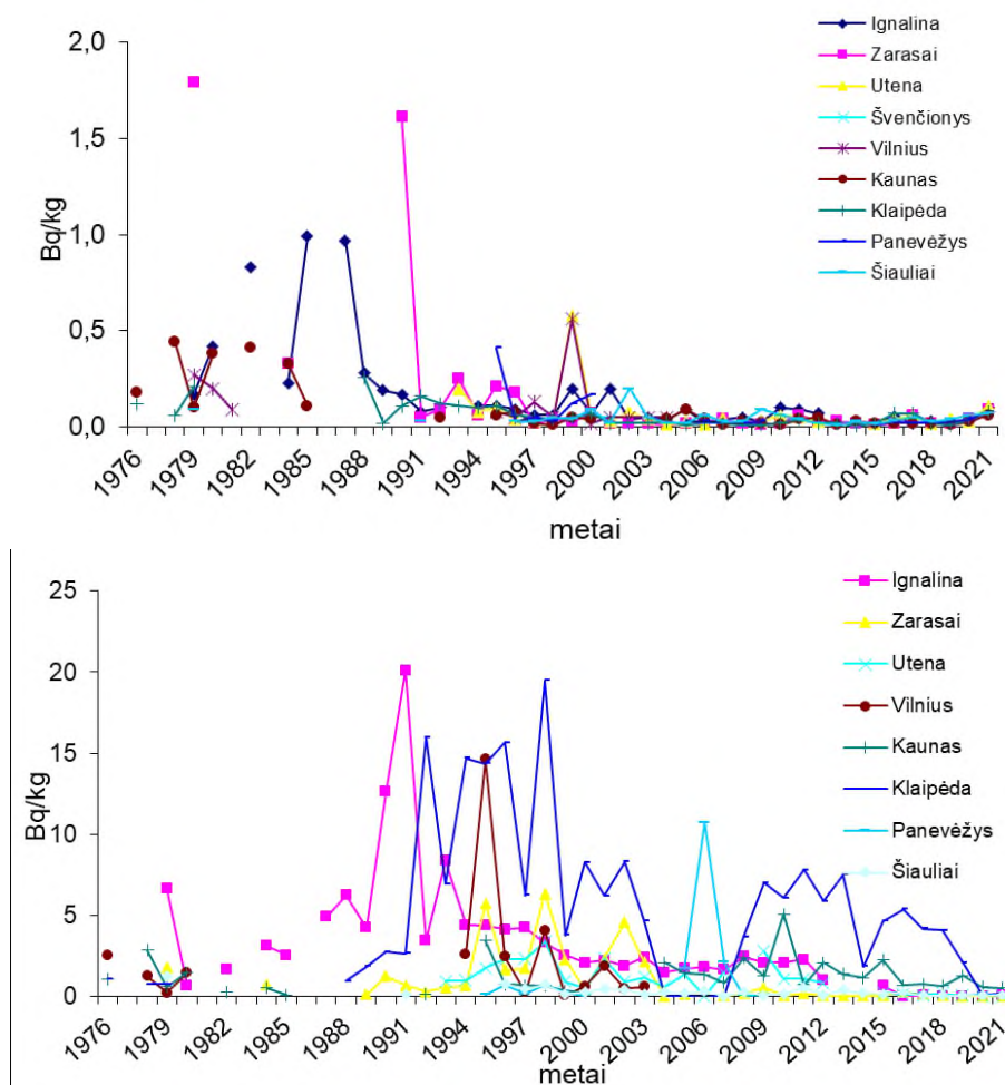
Pav. 3.5-3 Vidutinės metinės ^{90}\text{Sr} (viršuje) ir ^{137}\text{Cs} (apačioje) aktyvumo koncentracijos vertės žuvies mėginiuose, Bq/kg, 1976-2021 m. [3]
