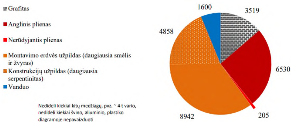
Pav. 2.4-2 Preliminarūs medžiagų kiekiai R3 zonoje (t, abu blokai kartu)
