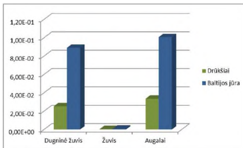
Pav. 3.5-2 Dozės galia ( \mu\text{Gy/val.} ) dėl ^{137}\text{Cs} [2]
