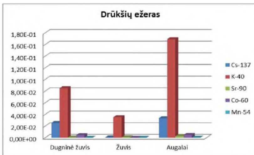
Pav. 3.5-1 Dozės galia ( \mu\text{Gy/val.} ) dėl įvairių radionuklidų [2]
